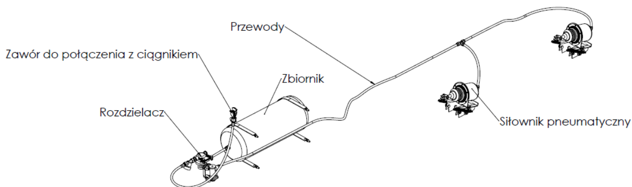
Rys.15 Schemat jednoobwodowej pneumatycznej instalacji hamulcowej
