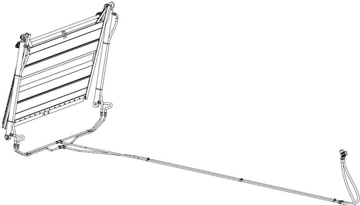
Rysunek 12 Instalacja hydrauliczna ściany tylnej.
