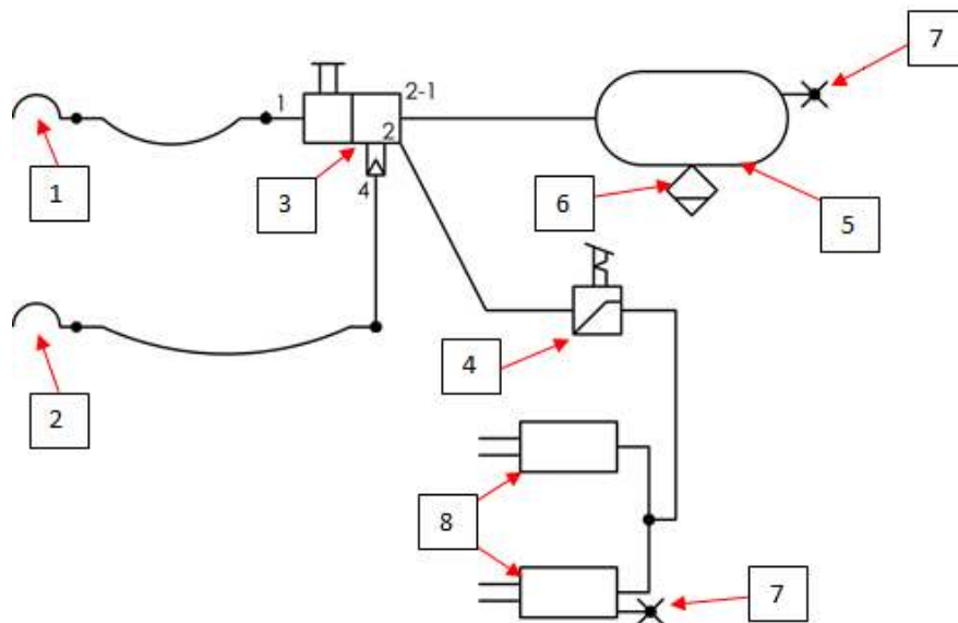
Rysunek 13. Schemat pneumatycznej instalacji hamulcowej
