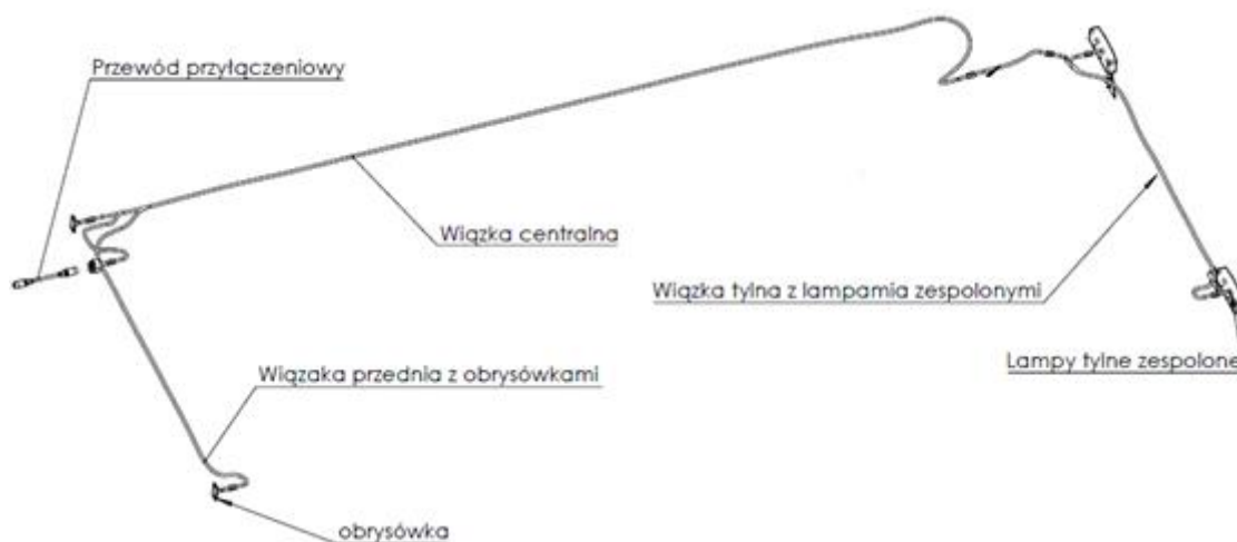
Rys. 17. Schemat instalacji elektrycznej rozrzutnika.
