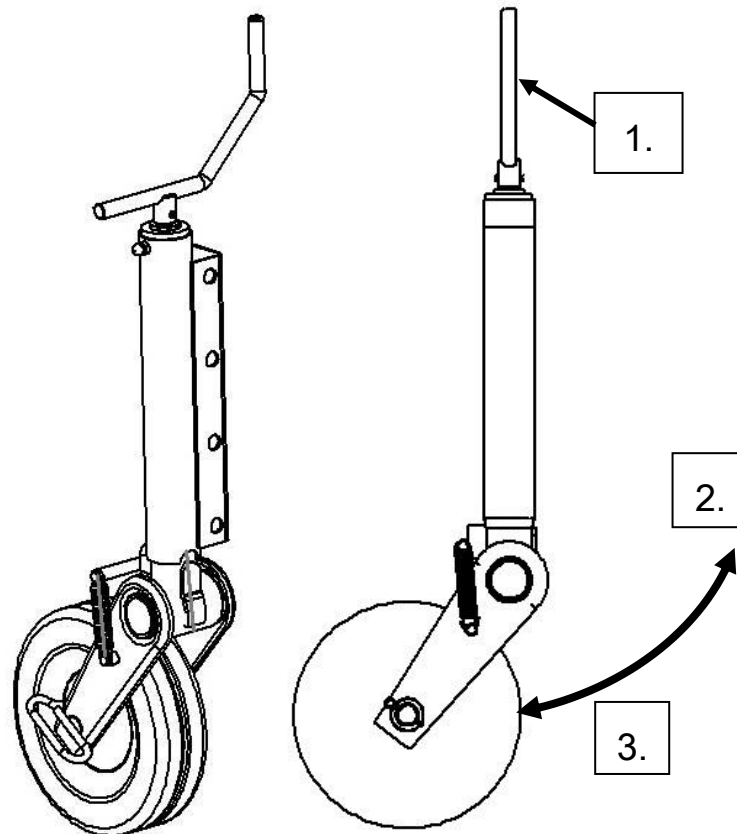
Rysunek 20. Regulowana podpora (od lewej: izometria, rzut z boku).
