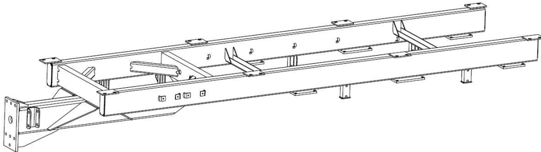
Rysunek 7. Rama dolna .
