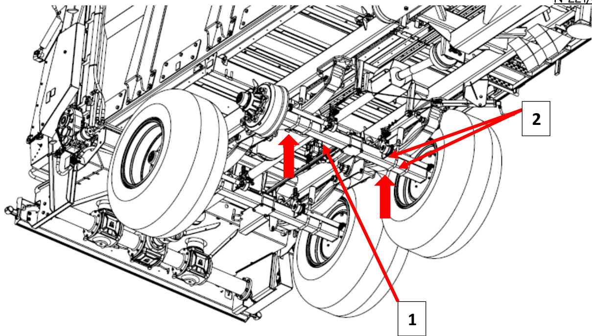
Rysunek 22. Punkt podparcia podnośnika
