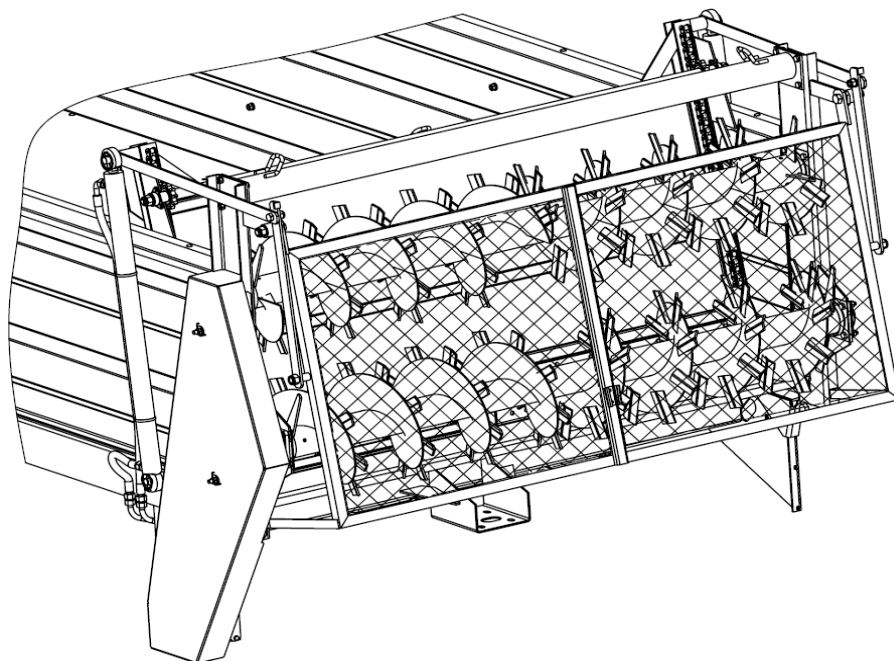
Rysunek 10 Adapter rozrzutnika
