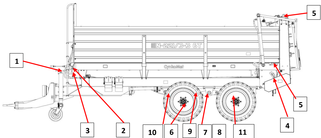
Rys. 26. Punkty smarowania N-221/3-3
