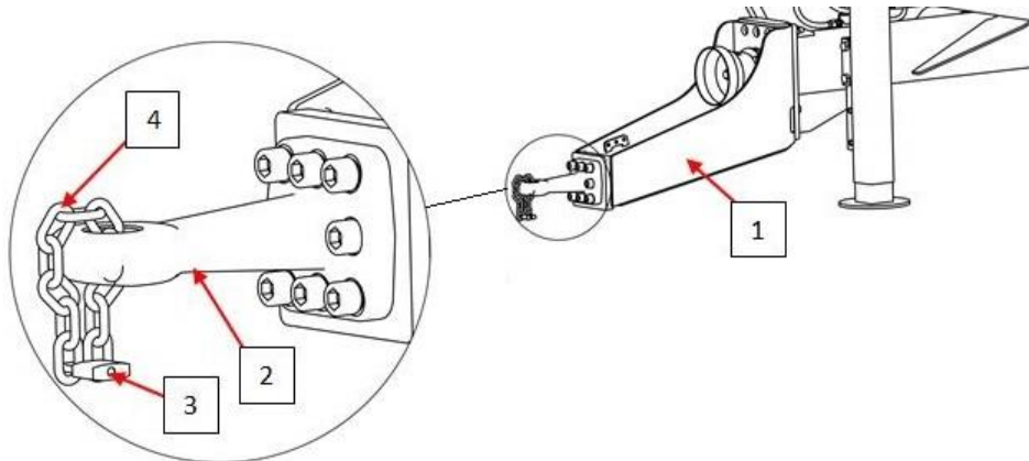
Rysunek 2. Zabezpieczenie maszyny przed nieupoważnionym użyciem.
