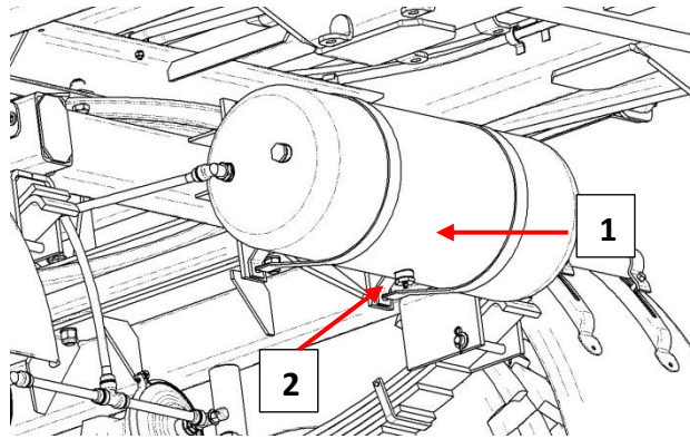
Rys. 24. Odwadnianie zbiornika powietrza
