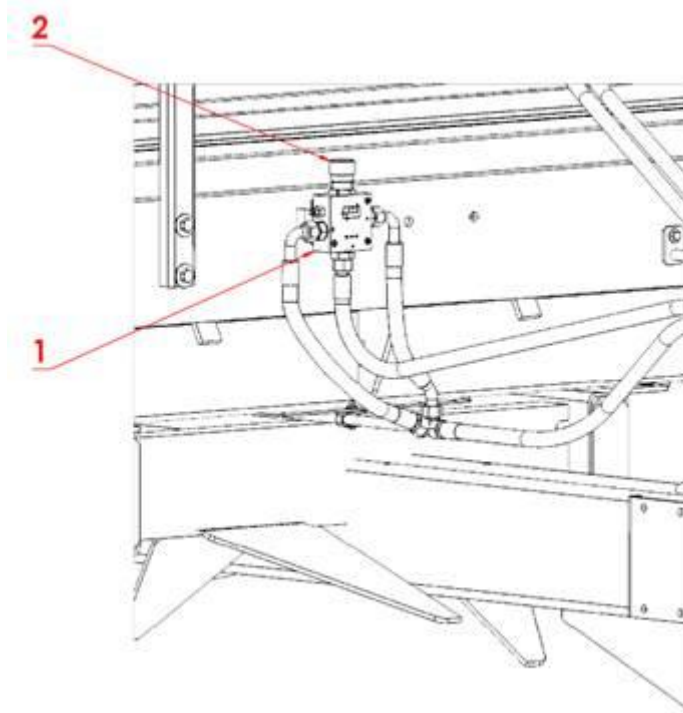
Rysunek 21. Regulacja prędkości przesuwu przenośnika podłogowego
