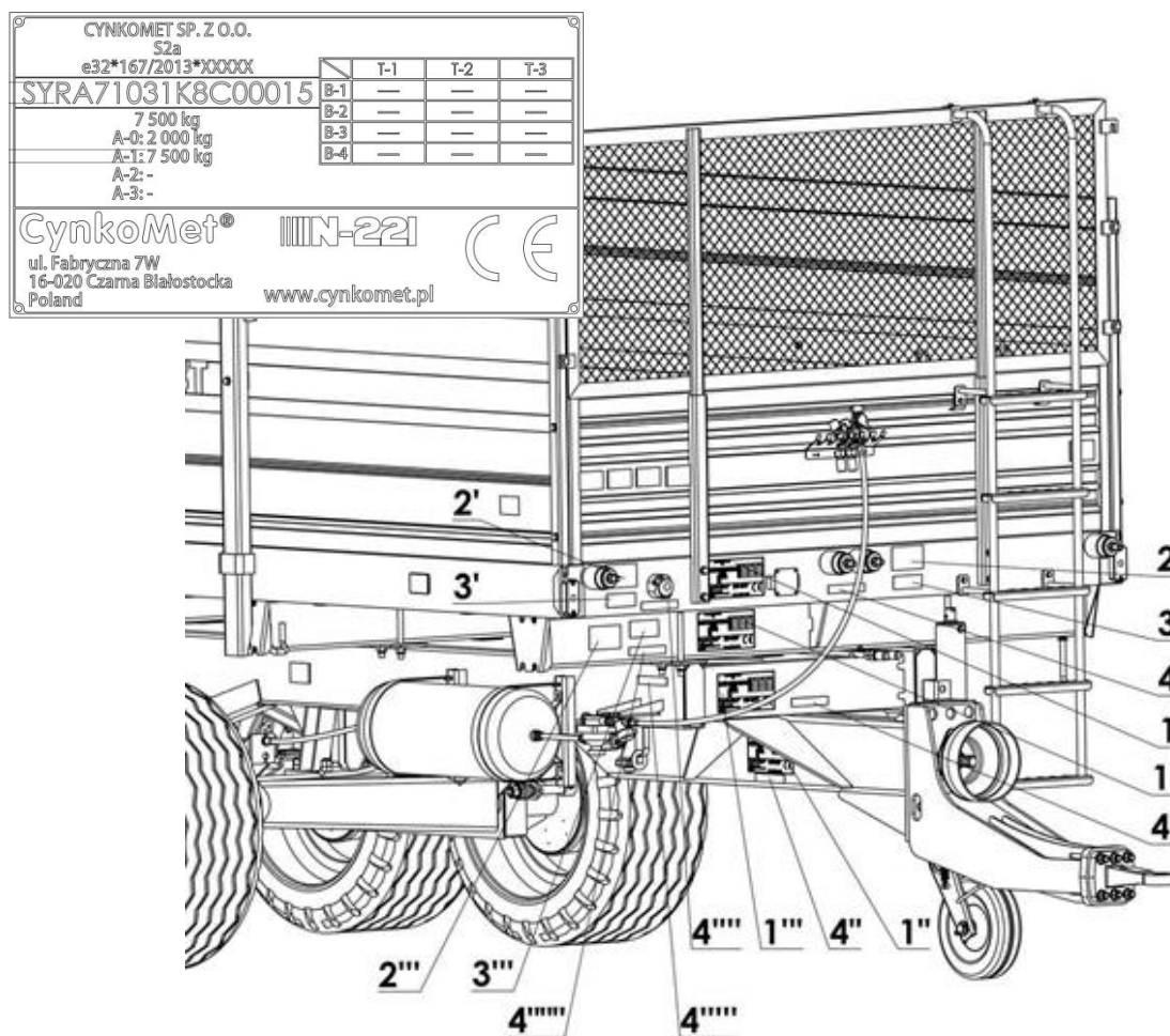
Rysunek 1. Możliwe miejsce umieszczenia tabliczki znamionowej i wybicia numeru fabrycznego 1 - tabliczka znamionowa, 2 - numer fabryczny, 3 - tabliczka znamionowa układu hamulcowego,
