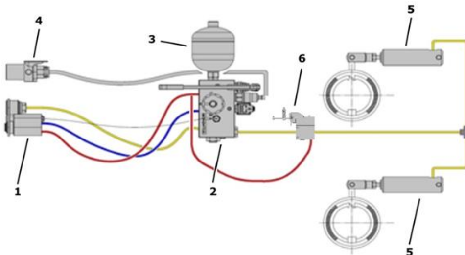
Rysunek 14. Schemat hydraulicznej instalacji hamulcowej.
